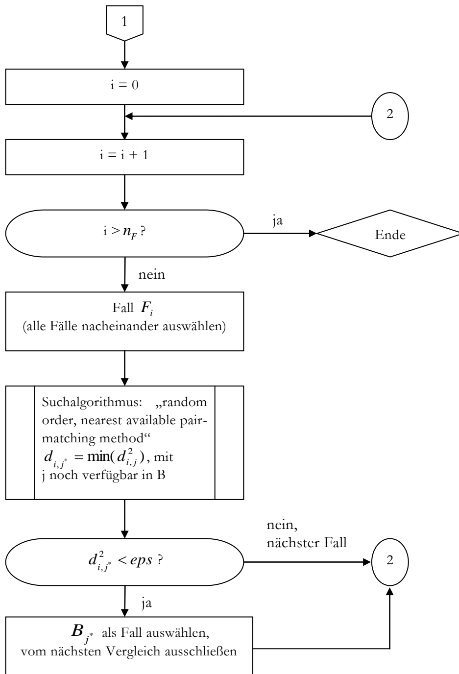
Abbildung 4 Algorithmus Matching
